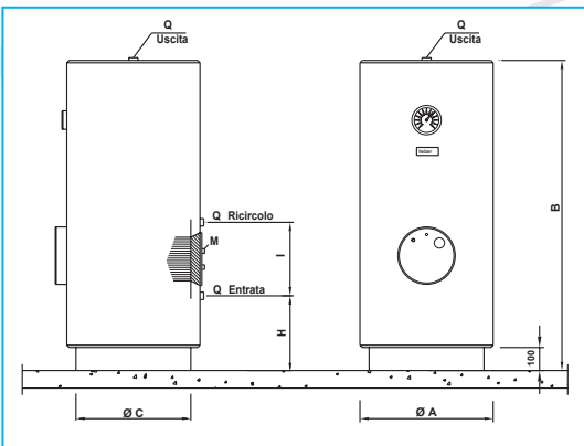
ET típus hőcserélőjének külső csatlakozásai
