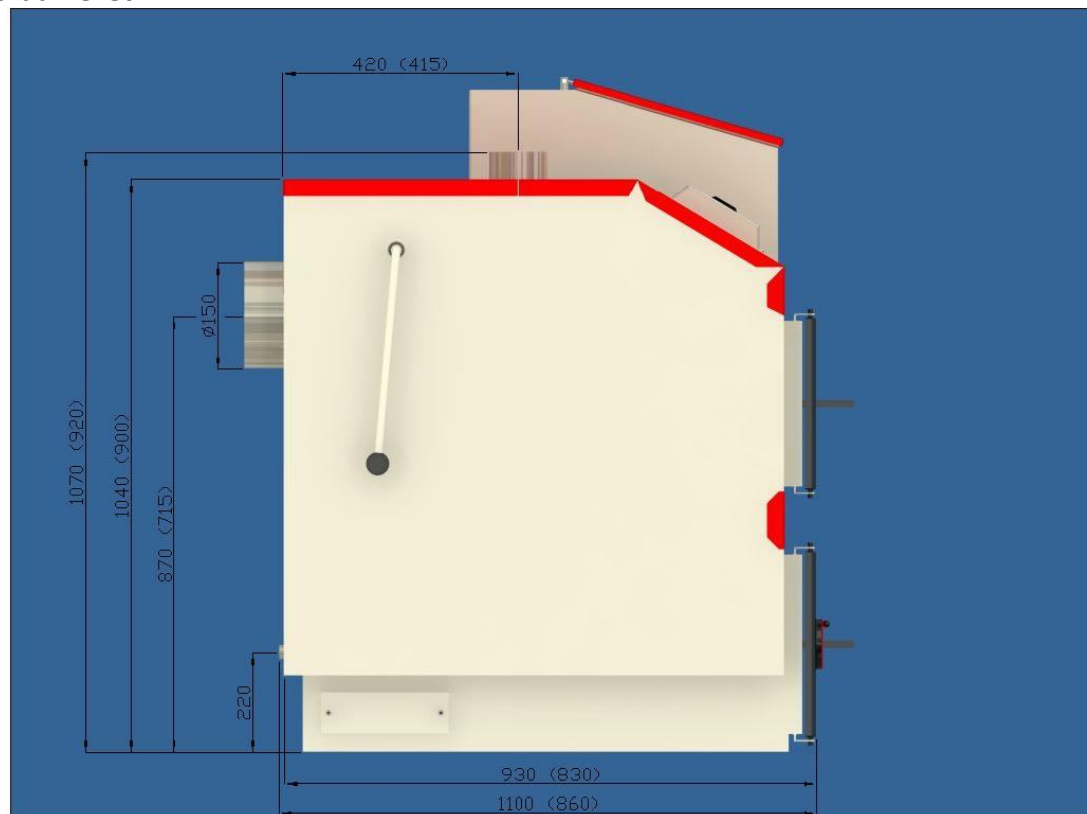
Oldalnézet
